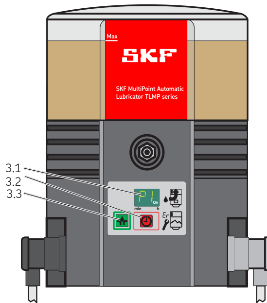
Folijas tastatūra ar displeju 5. att.
