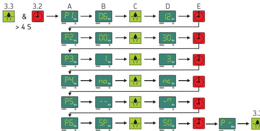
Рис. 10. Схема программирования
