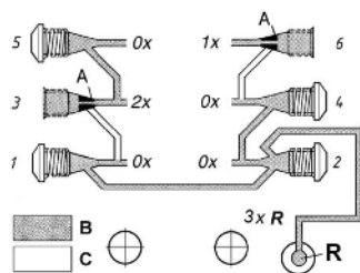
Výpuste 1, 2 a 4 vedené spät – obr. 4
