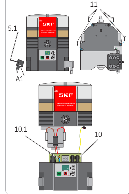
Kalvonäppäimistön vaihto, kuva 13
