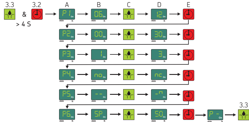
Programmēšanas shēma 10. att.
